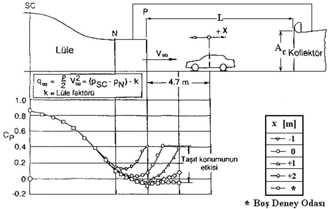
Şekil 3.8 10 m 2 'lik rüzgâr tünelinin içindeki modelin lüle çıkışına çok yakın yerleştirilmesi durumunda, N konumundaki statik basınç yükselmesi
