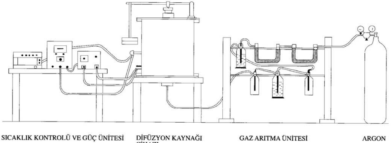
Şekil 1. Difüzyon kaynağı aparatı (şematik)
