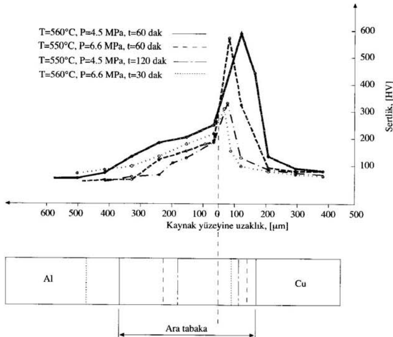
Şekil 2. Değişik kaynak şartlarında birleşme bölgesindeki mikrosertlik değişimleri
