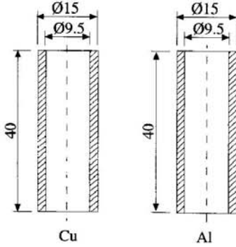
Şekil 8. Boru difüzyon kaynağı numuneleri
