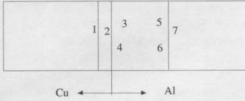
Şekil 4. EDS analiz bölgelerinin şematik gösterimi
